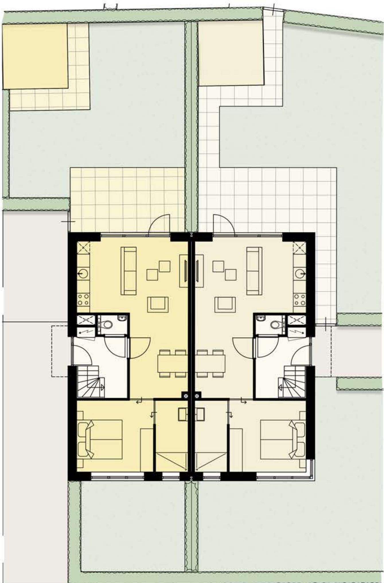
Begane grond levensloopbestendig
