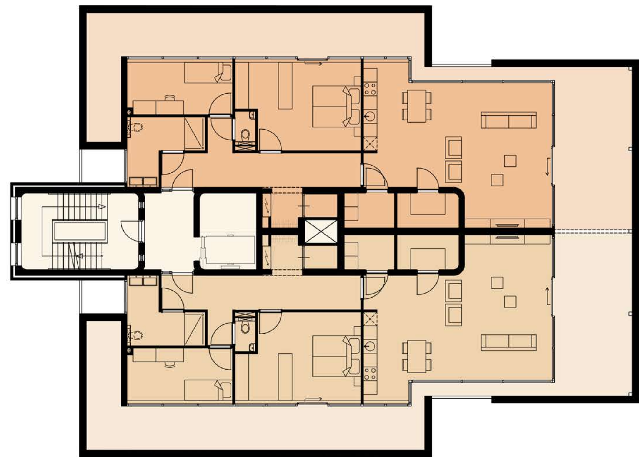
Verdieping 5
